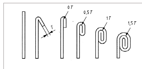
图6 - T-bends
