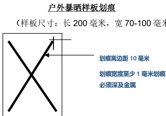
Figure 7 – 户外暴晒样板划痕
